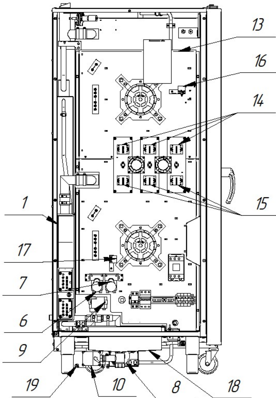
Рис.2б. Система водоснабжения, водоотведения и автоматической мойки (вид слева)
