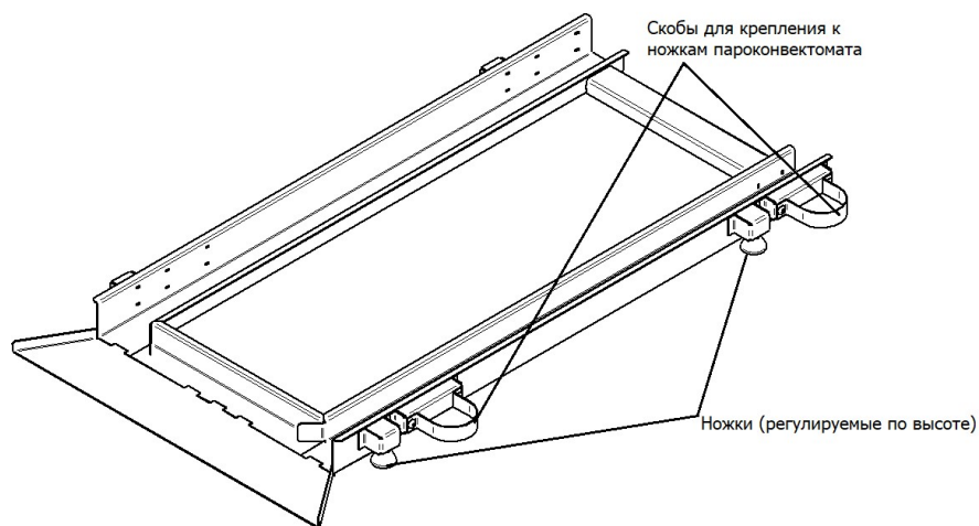
Подставка ПТП-20
