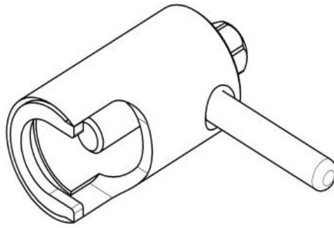
Рис. 13. Съемник крыльчатки.
